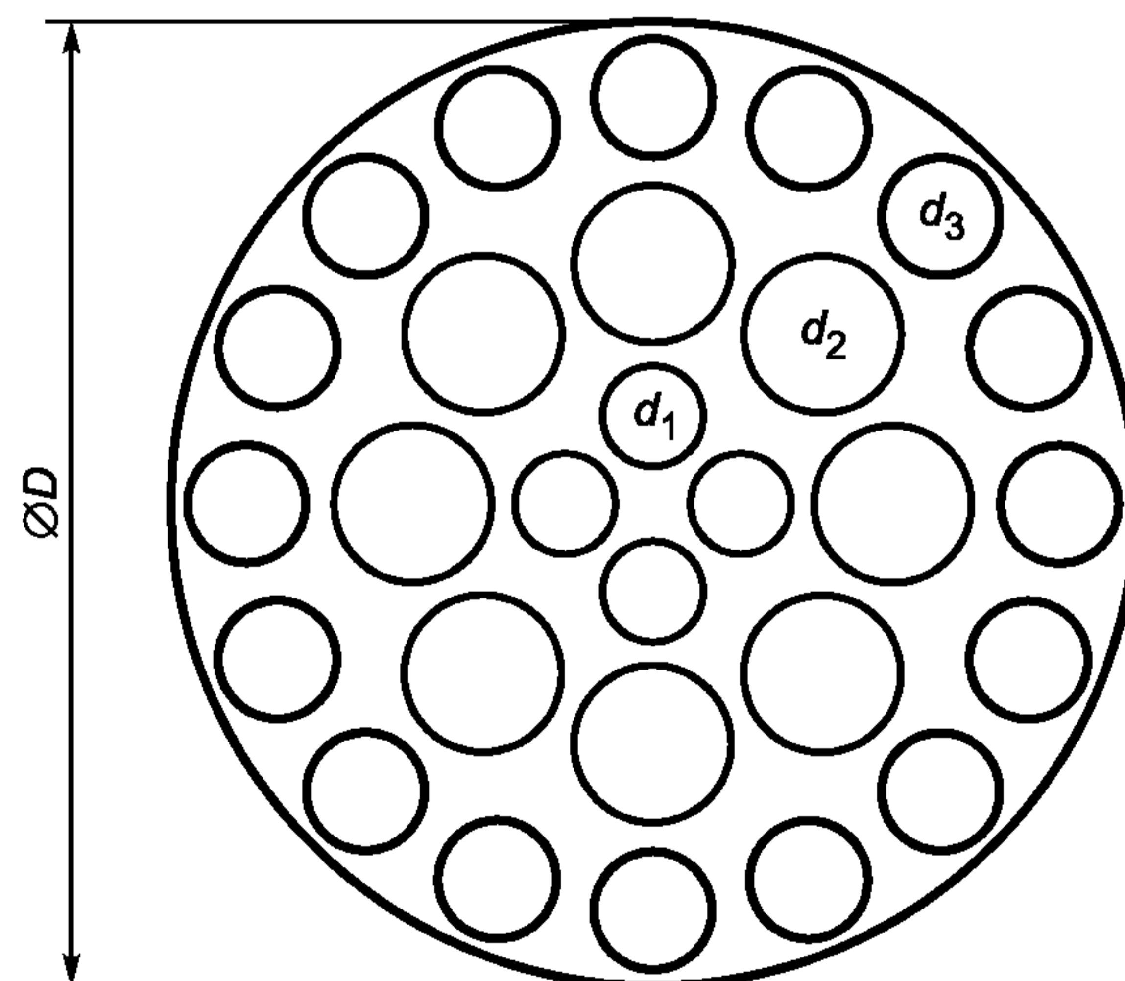
Рисунок В.2 — Выпрямитель потока
