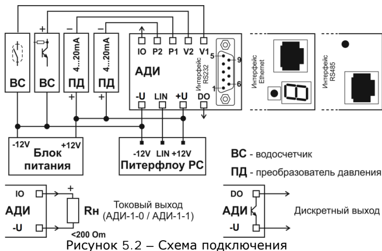
Рисунок 5.2 – Схема подключения
